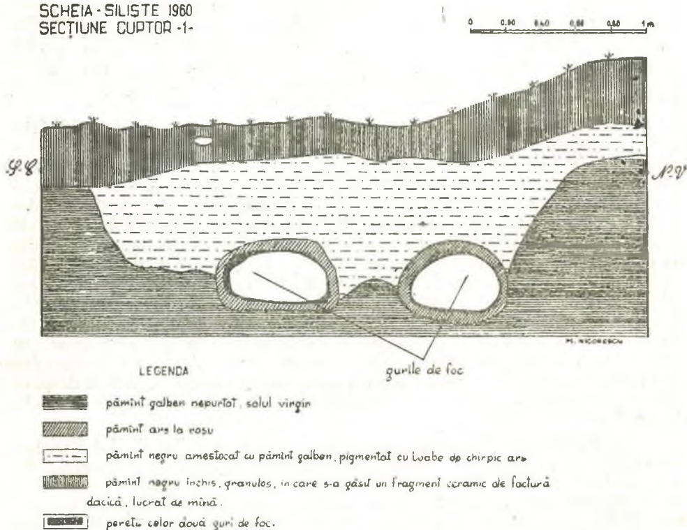
Fig. 2. — Secțiune prin cuptorul I.
