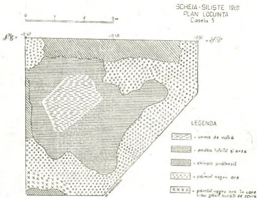
Fig. 1. — Planul locuinței descoperite în caseta 5.
