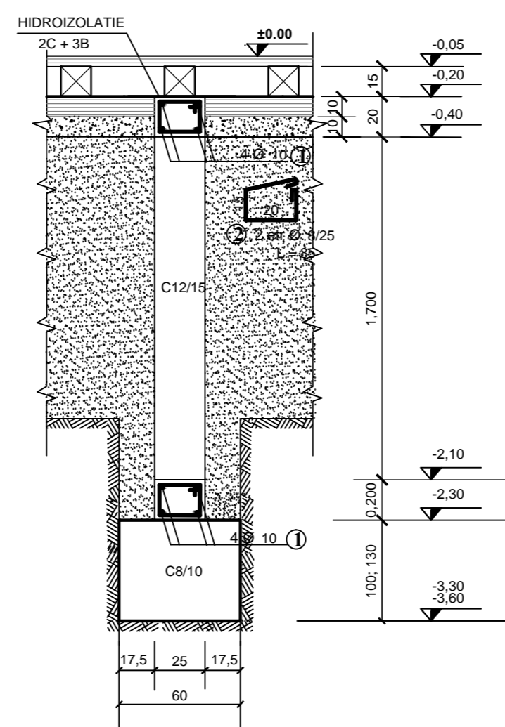
sectiune A - A
