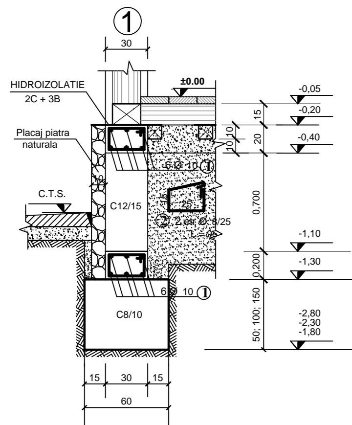
Detalii contrafort (4 buc.)
