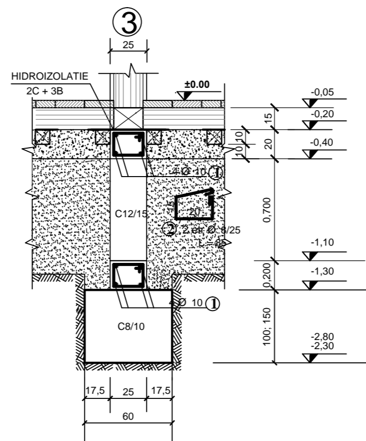
sectiune A - A
