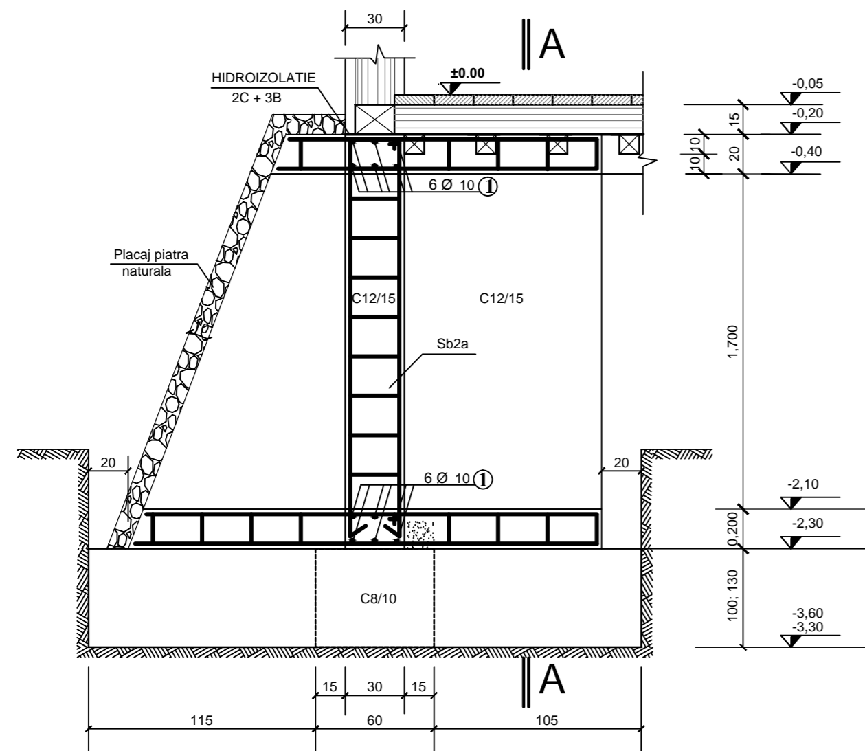
Detalii contrafort (4 buc.)
