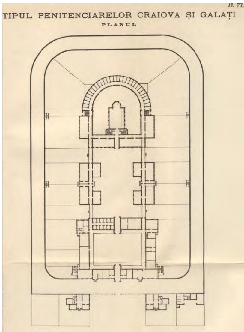
Fig. 9. Planul penitenciarelor Craiova și Galați 54
